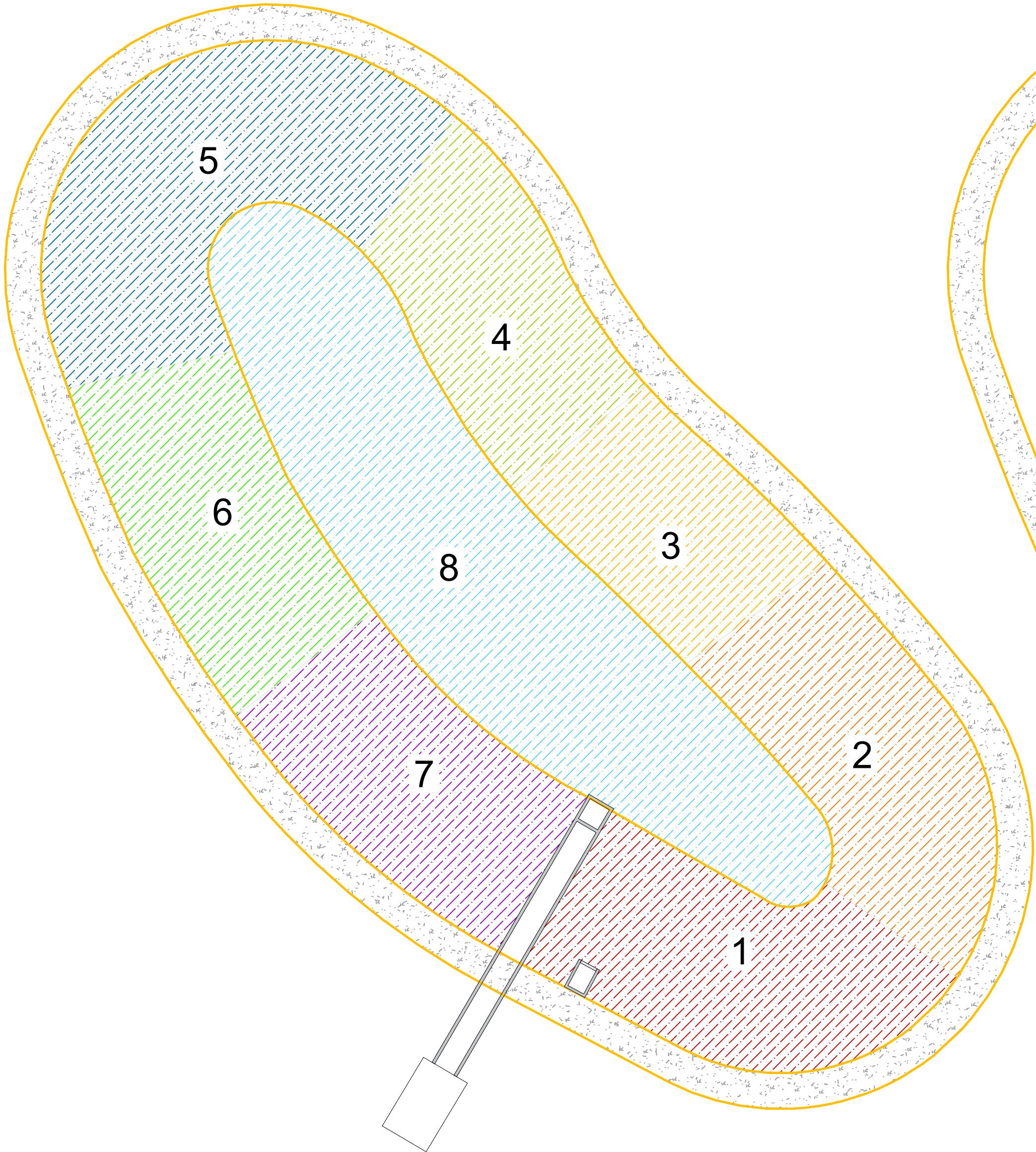
SCHEMA DRENAGGI PER MONITORAGGIO INTEGRITA' MANTO IMPERMEABILE
